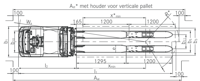
Bovenaanzicht OPX-L 16
