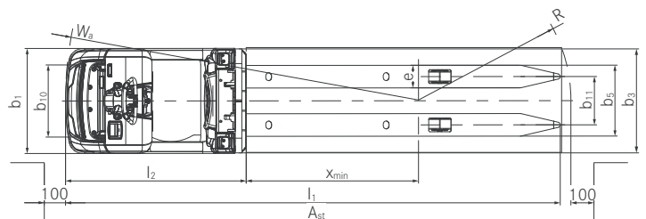
Bovenaanzicht OPX-L 20 S
