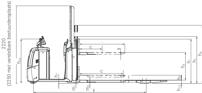
Zijaanzicht OPX-L 20
