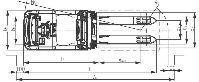
Bovenaanzicht OPX-D 20
